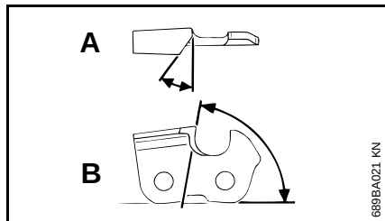
A Ángulo de afilado
