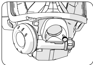
Abb. 1 Aktivierter Überdruck
